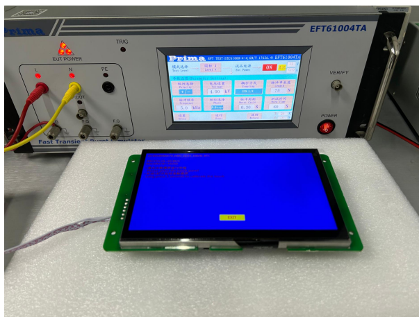
图 4-3 EFT 测试图
