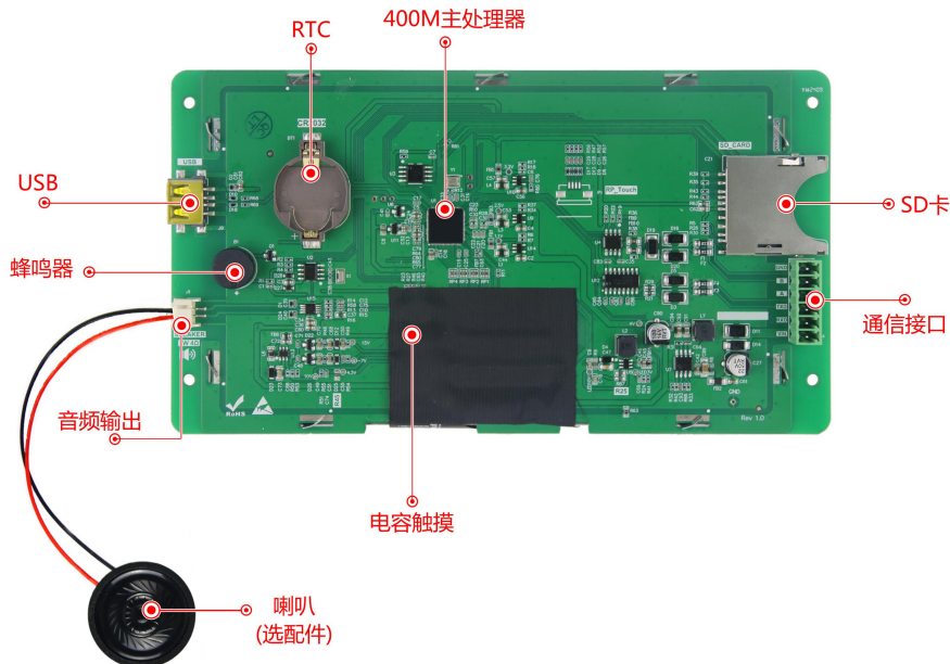
图 1-2 硬件配置图
