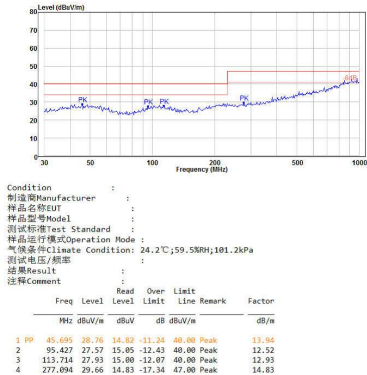
图 4-5 RE 测试水平方向
