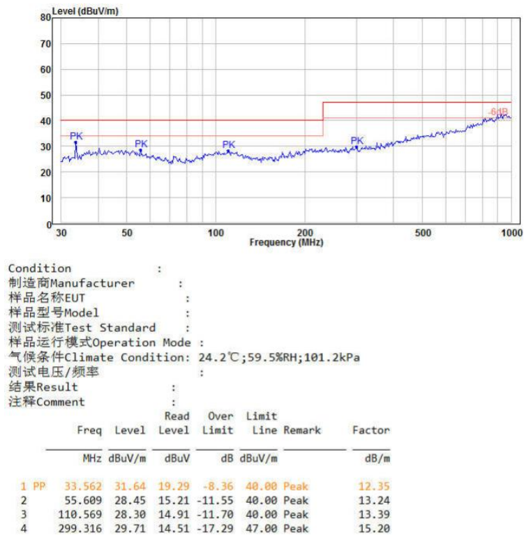
图 4-6 RE 测试垂直方向
