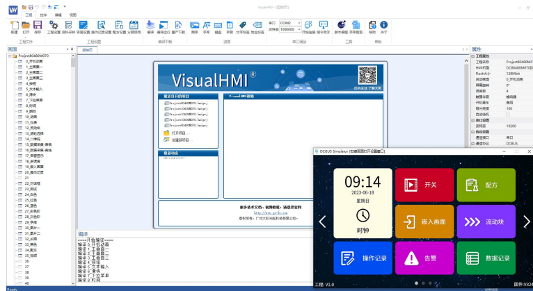
图 6-1 VisualHMI 主界面
